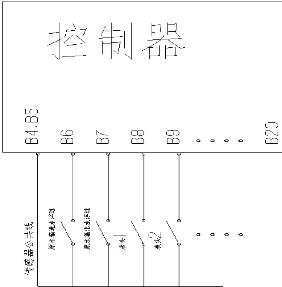
传感器、浮球控制端接线图(B4-B20)
