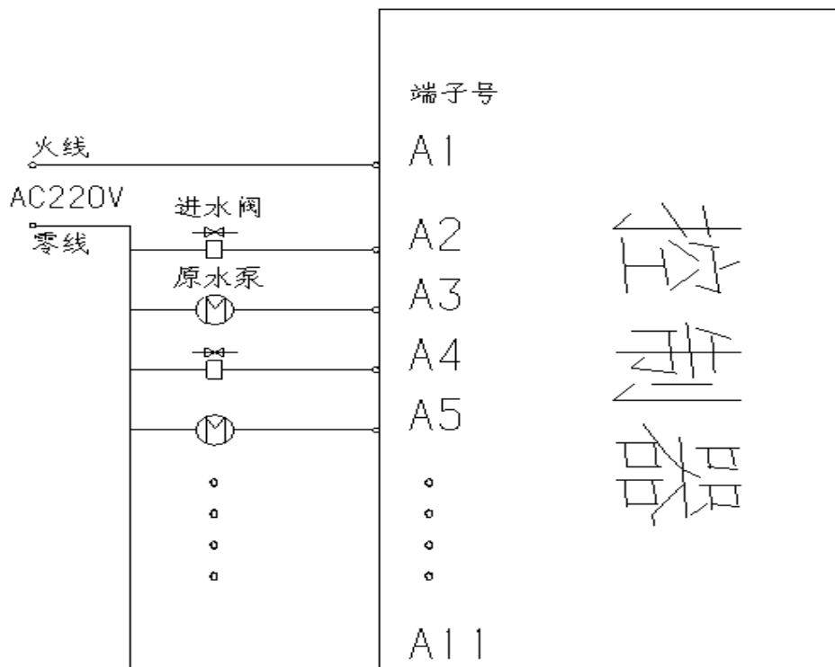
电磁阀、接触器控制端接线图(A1-A11)
